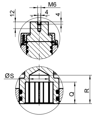
DETALLE EJE
