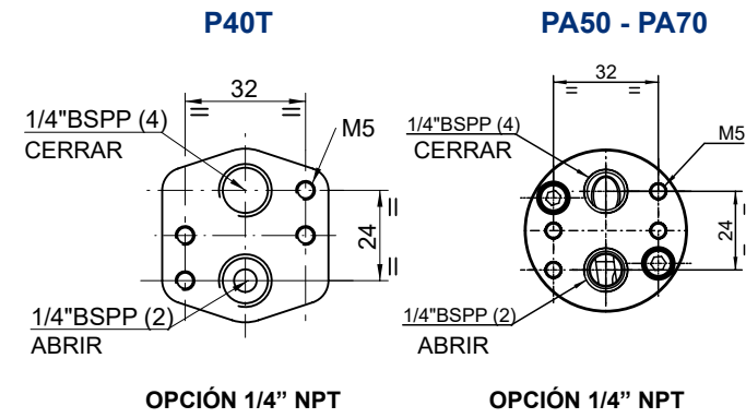
DETALLE EJE
