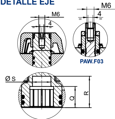
DETALLE EJE
