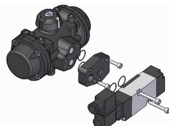
MONTAJE E.V. 3/2 VIAS (EV701) A ACTUADOR S.E. 3/2 WAYS S.V. (EV-701) MOUNTING TO S.R. ACTUATOR
