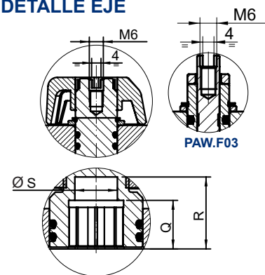
DETALLE EJE
