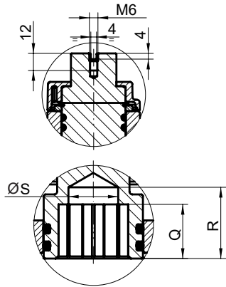
DETALLE EJE
