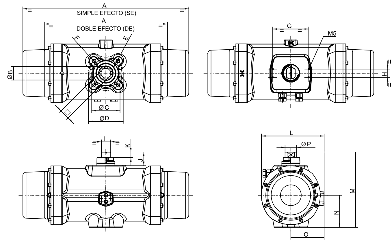
DIMENSIONES P40T - PA70
