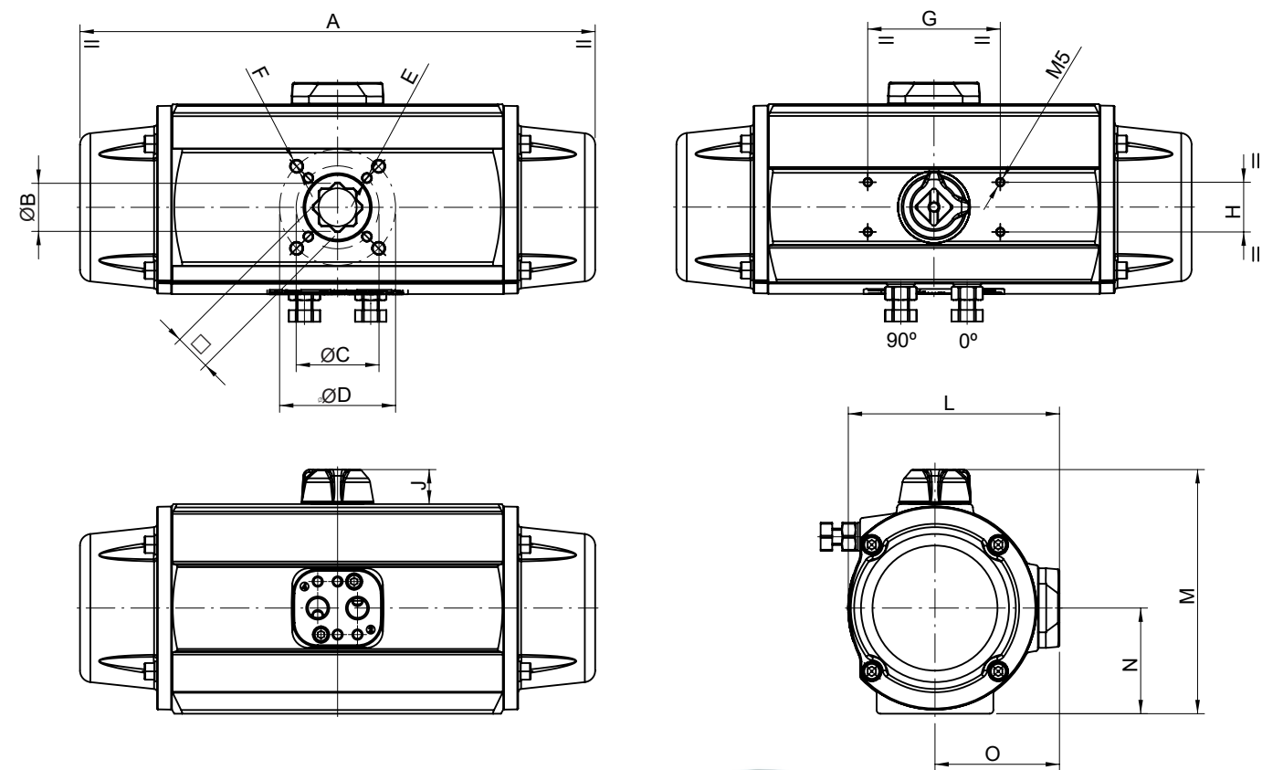
DIMENSIONES PAW.F03 - PA30
