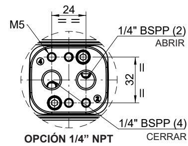
CONEXIÓN NEUMÁTICA NAMUR
