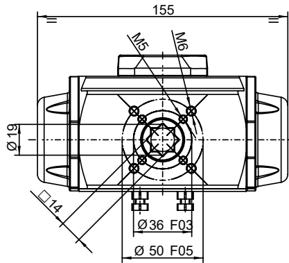
VISTA: DETALLE EJE VIEW: SHAFT DETAIL
